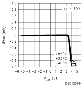
dV_{OS} vs V_{CM}
