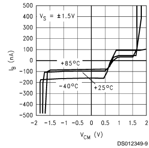
I_{bias} vs V_{CM}
