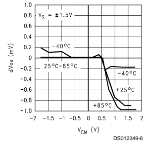
dV_{OS} vs V_{CM}
