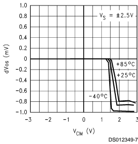
dV_{OS} vs V_{CM}
