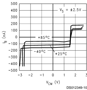
I_{bias} vs V_{CM}
