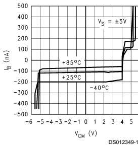
I_{bias} vs V_{CM}
