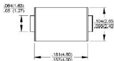
DO-214AC (SMA)
