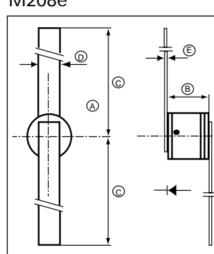
M208e C_b=0.12pF
