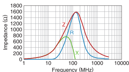
MMZ1608A222BTA00
