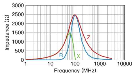
MMZ1608Q331BTA00
