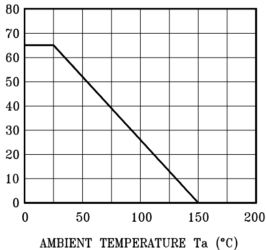
P_C - T_a
