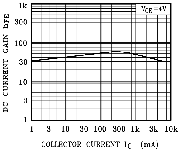
h_{FE} - I_C
