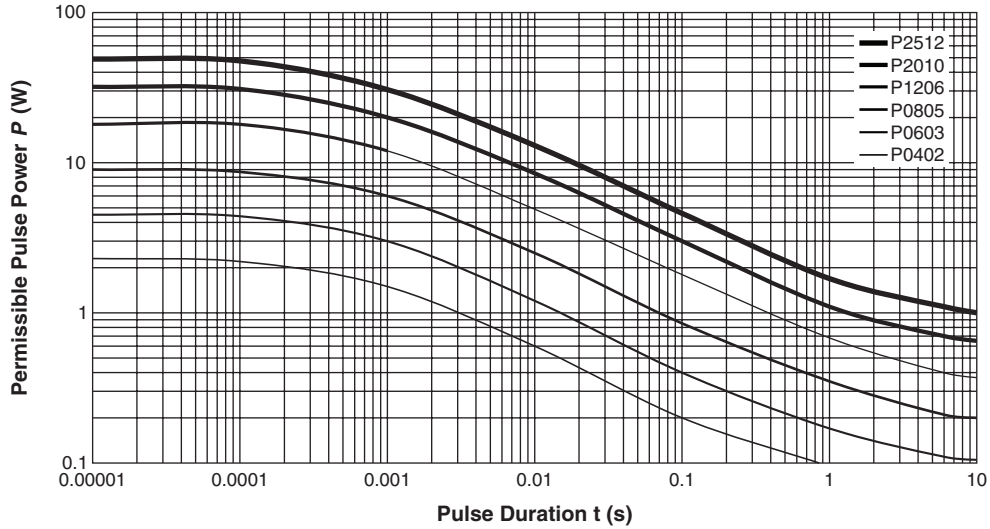
Maximum permissible pulse load P_i max.
