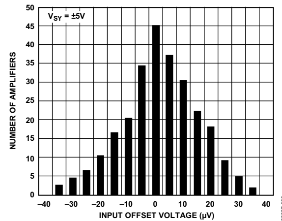
图30. 输入失调电压分布图
