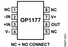
图2. 8引脚SOIC_N (R后级)
