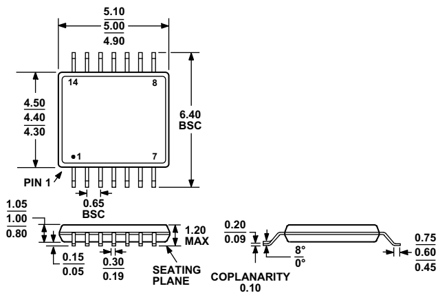
图72. 14引脚超薄紧缩小型封装[TSSOP] (RU-14)
