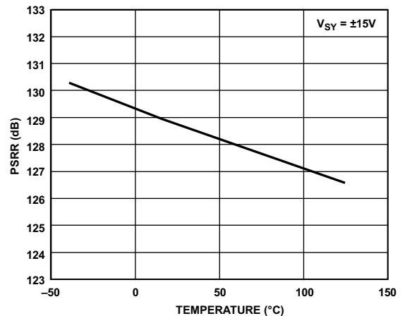
图29. PSRR与温度的关系
