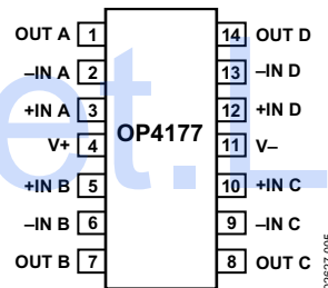
图5. 14引脚SOIC_N (R后级)
