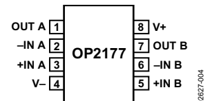
图4. 8引脚SOIC_N (R后级)
