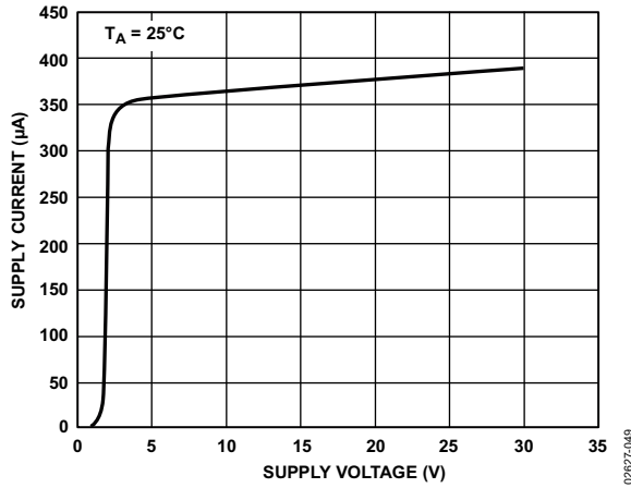
图49. 电源电流与电源电压的关系
