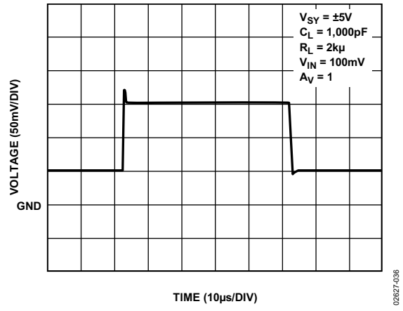
图36. 小信号瞬态响应
