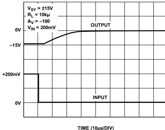
图18. 正过压恢复时间
