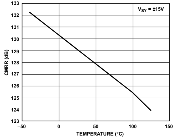
图28. CMRR与温度的关系
