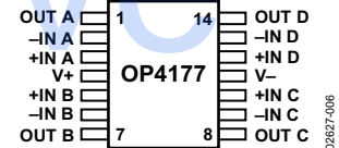
图6. 14引脚TSSOP (RU后级)
