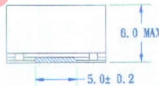
俯视图
