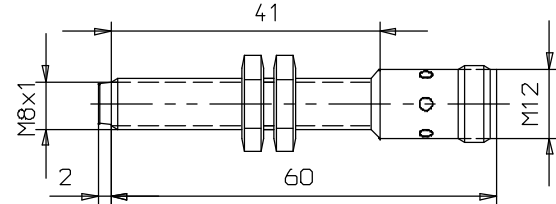
E2EL-X2M□-M1L
