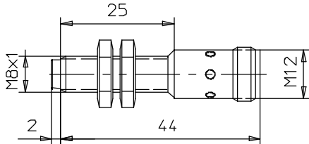
E2EL-X2M□-M1
