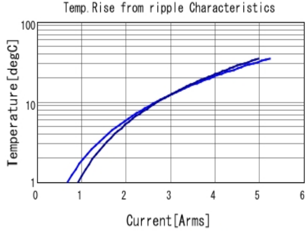
GRM219R6YA475MA73 Temp. rise ■ 500kHz ■ 1MHz
