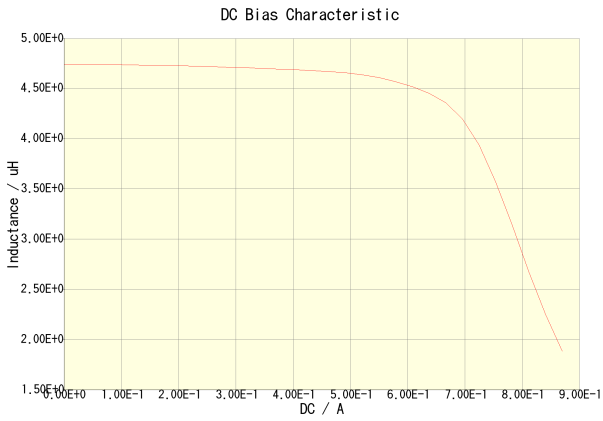
NLCV32T-4R7M-PF(Amb. Temp. = 20degC)
