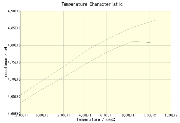
NLCV32T-4R7M-PF(DC = 0A)
